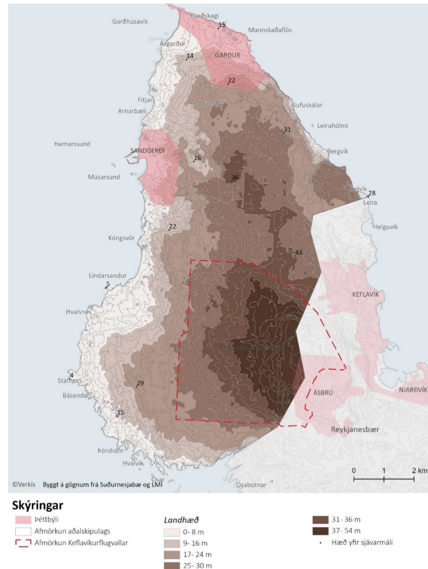
Mynd 10 Landslag og hæð lands í Suðurnesjabæ.
